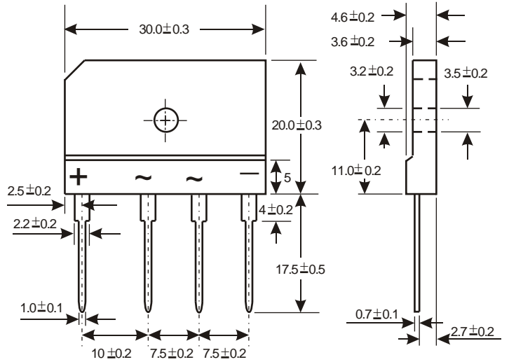
RS-20M
